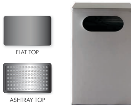
SRT382375 (FT) SRT382375 (AT) 380(L) X 230(D) X 750(H) (mm) 52 LITRES
